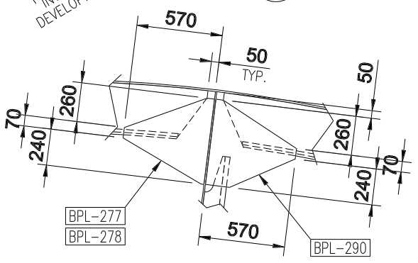
2 DETAIL Scale: NTS
