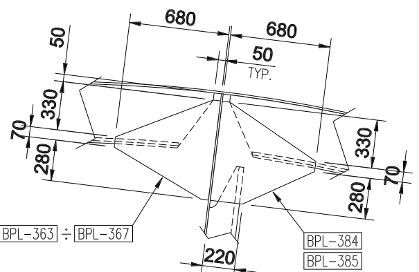
3 DETAIL Scale: NTS
